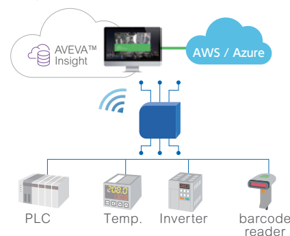
STM6000 Edge Box HMI
